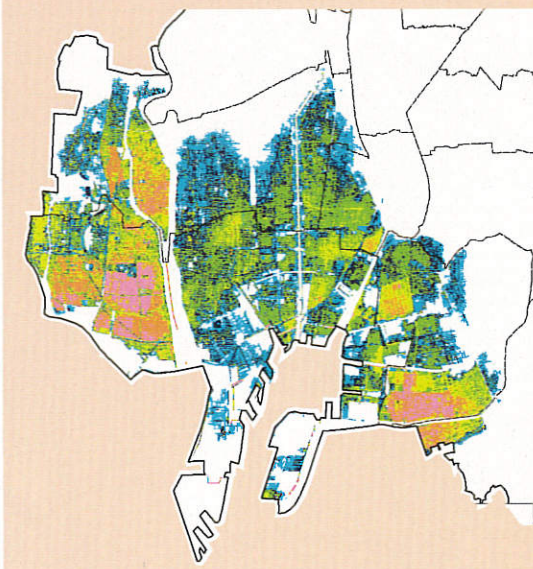
過去の地震を考慮した最大クラス
