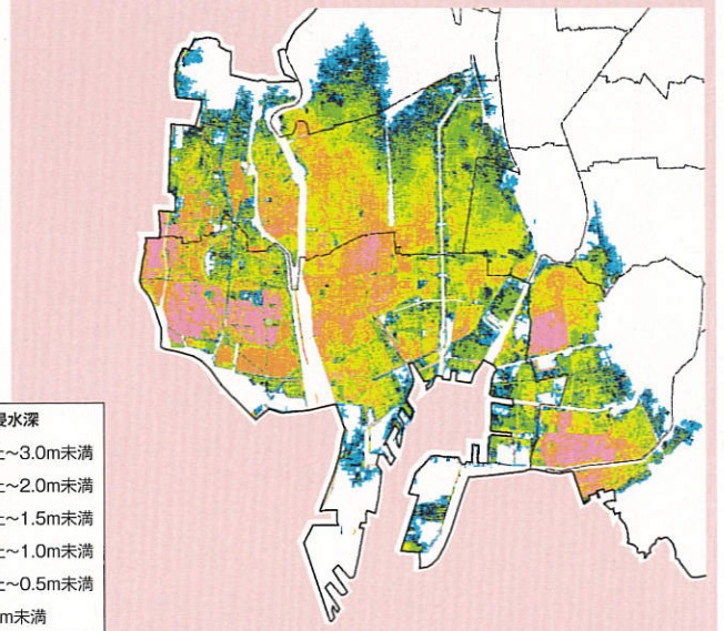
あらゆる可能性を考慮した最大クラス
